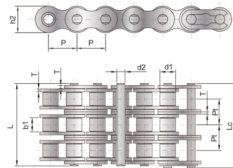
加重系列滚子链 Heavy duty series roller chain
