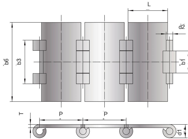
平顶链 Flat top chain
