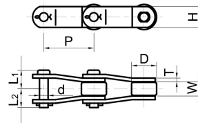
型式 9 Type 9 Chain
