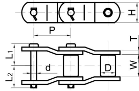
型式 8 Type 8 Chain
