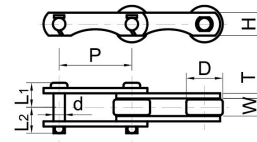
型式 12 Type 12 Chain
