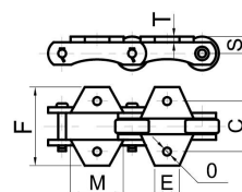
K1附件 K1 Attachment
