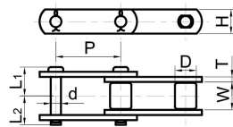
型式 10 Type 10 Chain
