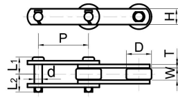
型式 11 Type 11 Chain
